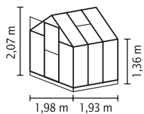
TRITON 3800
