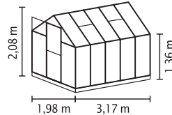
TRITON 6200
