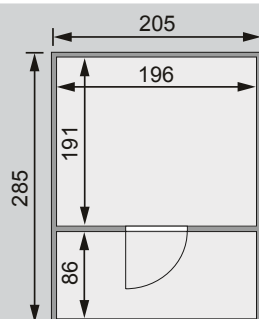
Außen-/Innenmaße (in cm)
