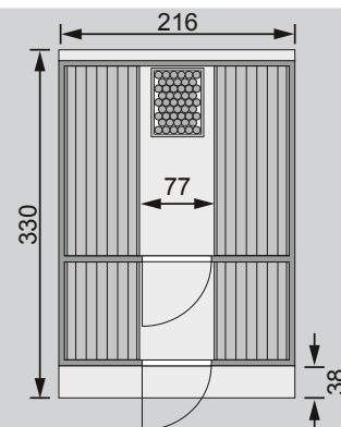
Dachstand / Innenaufteilung (in cm)
